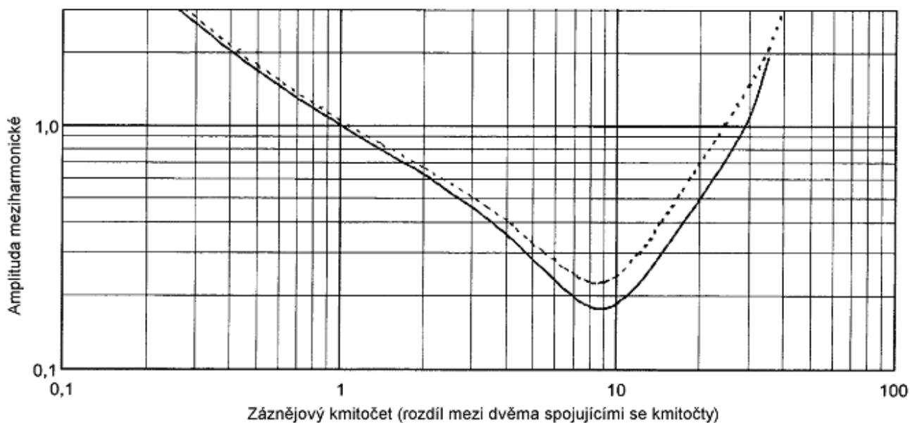
Obrázek 1 – Kompatibilní úrovně pro meziharmonické (Odezva flikrmetru pro P_{st} = 1 s ohledem na žárovky 60 W)
